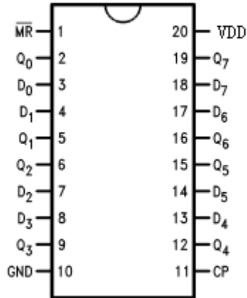
图 4-1 B54AC273RH 引脚排列图
