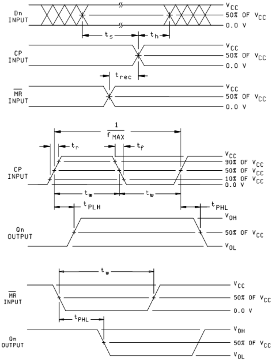
图 6-1 器件开关参数波形图
