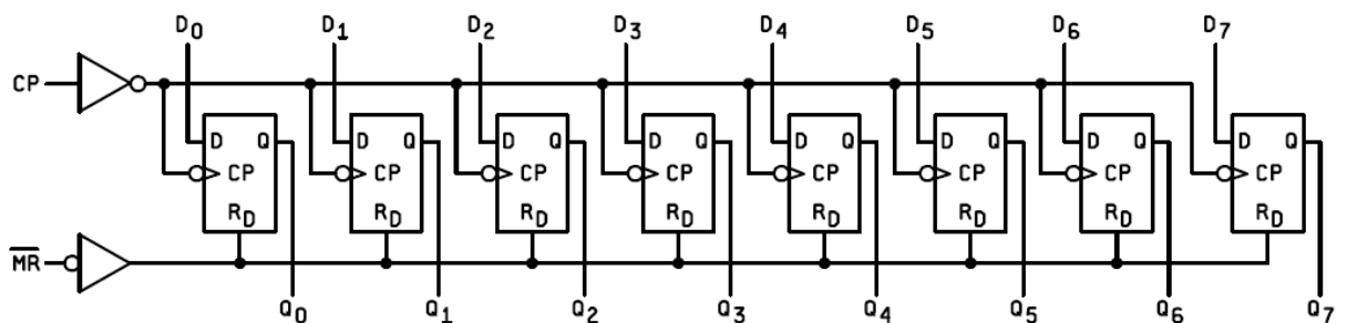
图 3-1 B54AC273RH 结构图
